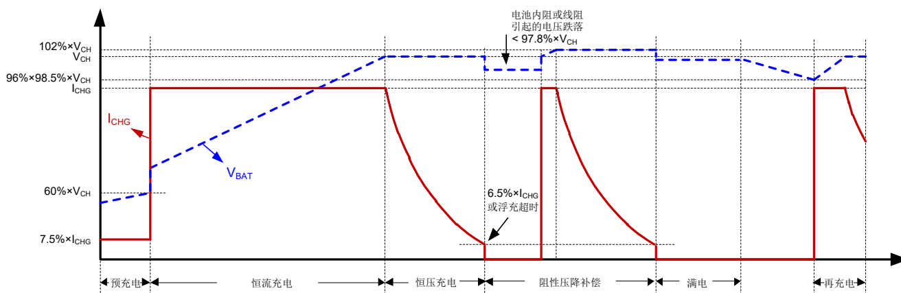
图 5. SGM40560A 充电周期示意图 (阻性压降大于 2.2\% \times V_{CH} )
