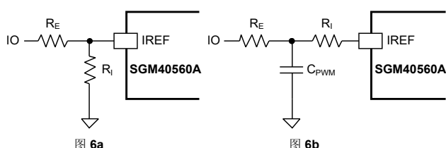
图 6. 两种控制充电电流的方式
