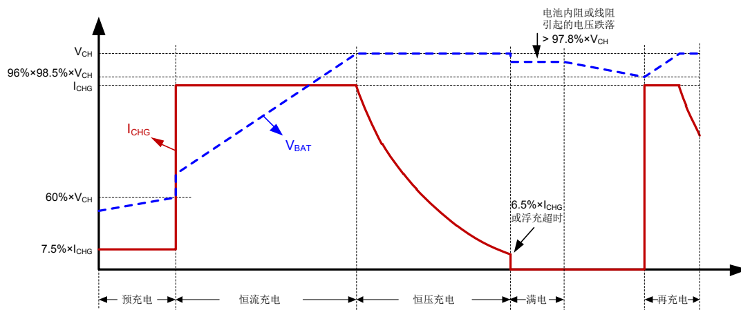
图 4. SGM40560A 充电周期示意图 (阻性压降小于 2.2\% \times V_{CH} )
